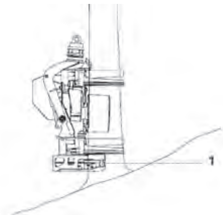
Obr. 43 Správná výška řezu (1) při kácení ve svahu
