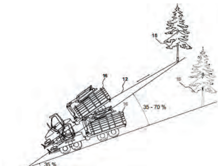
Obr. 60 Nasazení vyvážecího traktoru s trakčním navijákem
