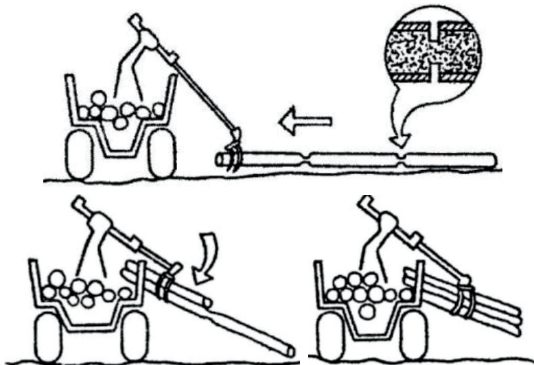
Obr. 45 „Nalámání“ sdruženého výřezu na ložnou plochu vyvážecího traktoru
