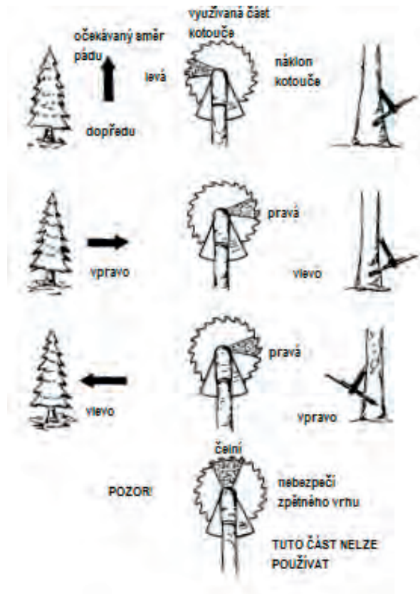
Obr. 38 Usměrnění pádu stromů při práci s křovinořezem
