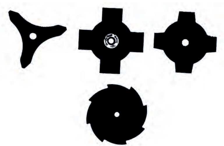
Obr. 35 Kovové pracovní nástroje pro vyžínání bylinné vegetace a dřevinných nárostů do tloušťky max. 15 mm
