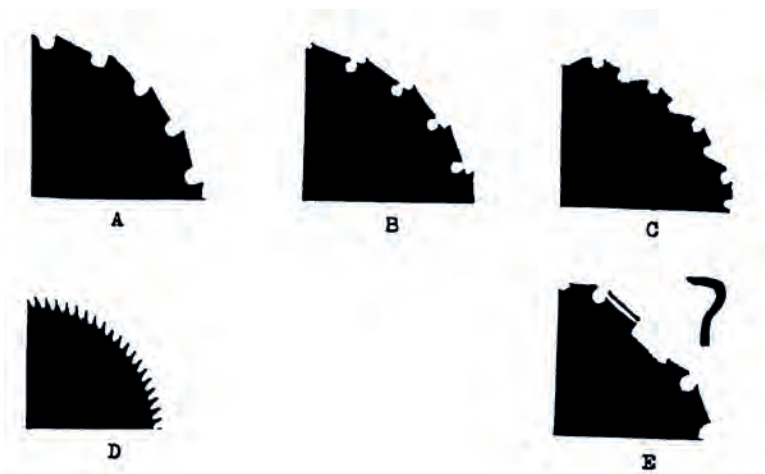
A, B – vlčí ozubení, C – vlčí ozubení s omezovacími patkami, D – trojúhelníkové ozubení, E – hoblovací ozubení
