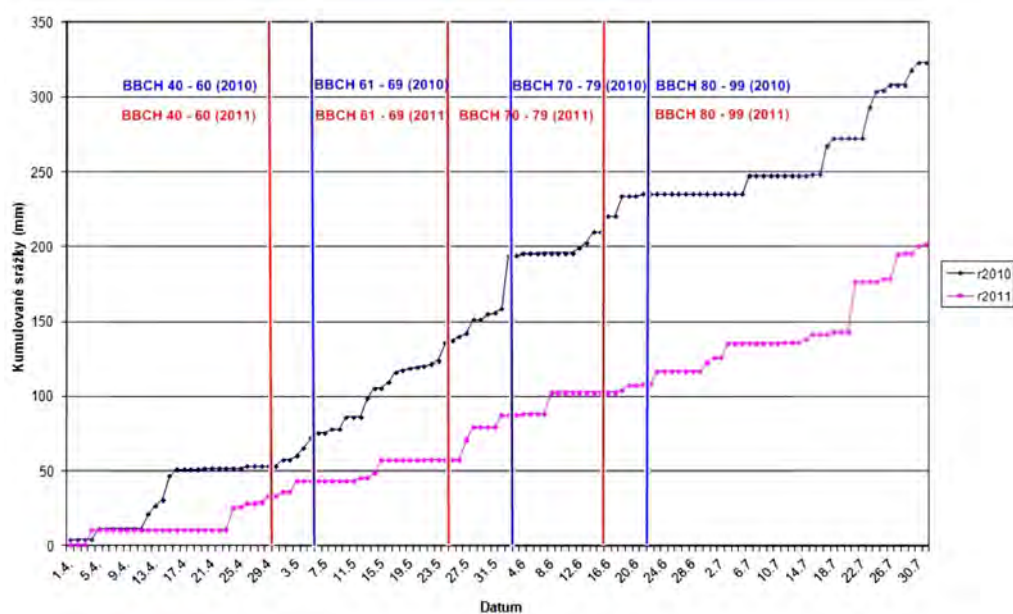
Obr. 4 Nahore: kumulované srážkové úhrny pro vyjádření dynamiky srážek a snadnou identifikaci bezsrážkových období a objemová vlhkost půdy během jednoho období (leden–červenec); dole: kumulované srážkové úhrny na jedné lokalitě během dvou let a jejich rozdělení do období dle markantních růstových fází řepky olejně v konkrétním roce, umožňující přehledné porovnání ročníků z pohledu srážkové činnosti
