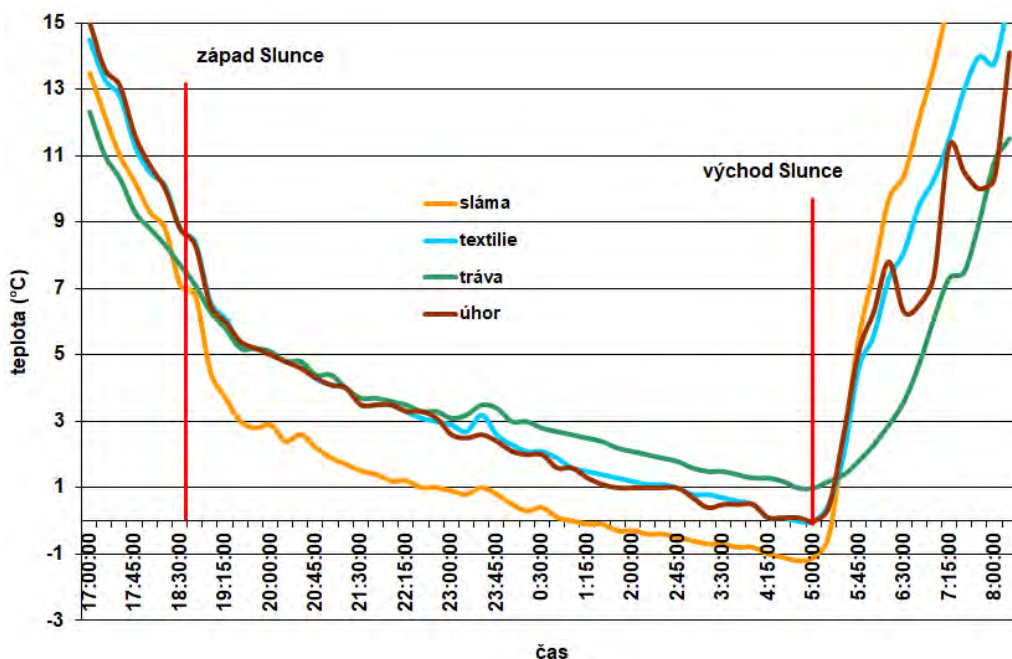
Obr. 18 Průběh teplot ve dnech 17.–18. 4. nad jednotlivými povrchy
