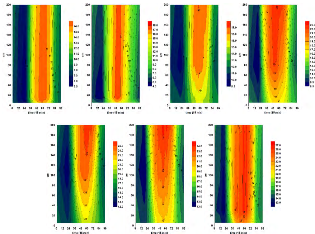
Obr. 19 Průměrné hodnoty teploty vzduchu (°C) ve vertikálním profilu porostu pšenice. Každý nomogram ukazuje virtuální průměrný den období, získaný zpřůměrováním hodnot za celé období. Na horizontální ose je uveden čas – 24hodinový den rozdělený po patnáctiminutových intervalech; na vertikální ose je výška měření. Zleva doprava: horní řada – období I. rok 1; období I. rok 2; období II. rok 1; období II. rok 2; dolní řada – období III. rok 1; období III. rok 2; období po polehnutí porostu ve druhém roce
