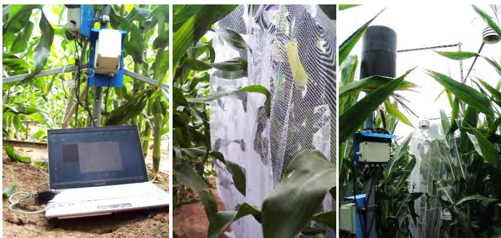
Obr. 30 Příklad monitoringu mikroklimatu porostu a půdního klimatu pro účely precizního specifikování nároků škodlivého činitele s využitím lapačů a izolátoru Zdroj: autoři
